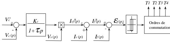
Figure 7 : Algorithme de commande.
