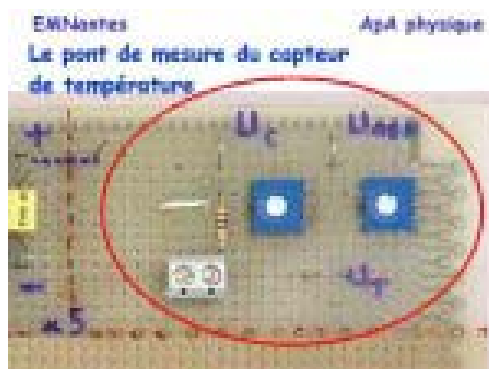
Fig. 4. Le pont de mesure du capteur de température.
