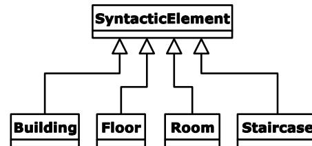
Fig.3. Hiérarchie des concepts syntaxiques
