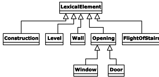
Fig.2. Hiérarchie des concepts lexicaux.
