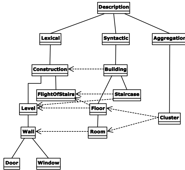
Fig.5. Les types de liaisons utilisées dans notre modèle : les traits pleins verticaux représentent les liaisons d'imbrication, tandis que les lignes pointillées horizontales représentent les liaisons de composition
